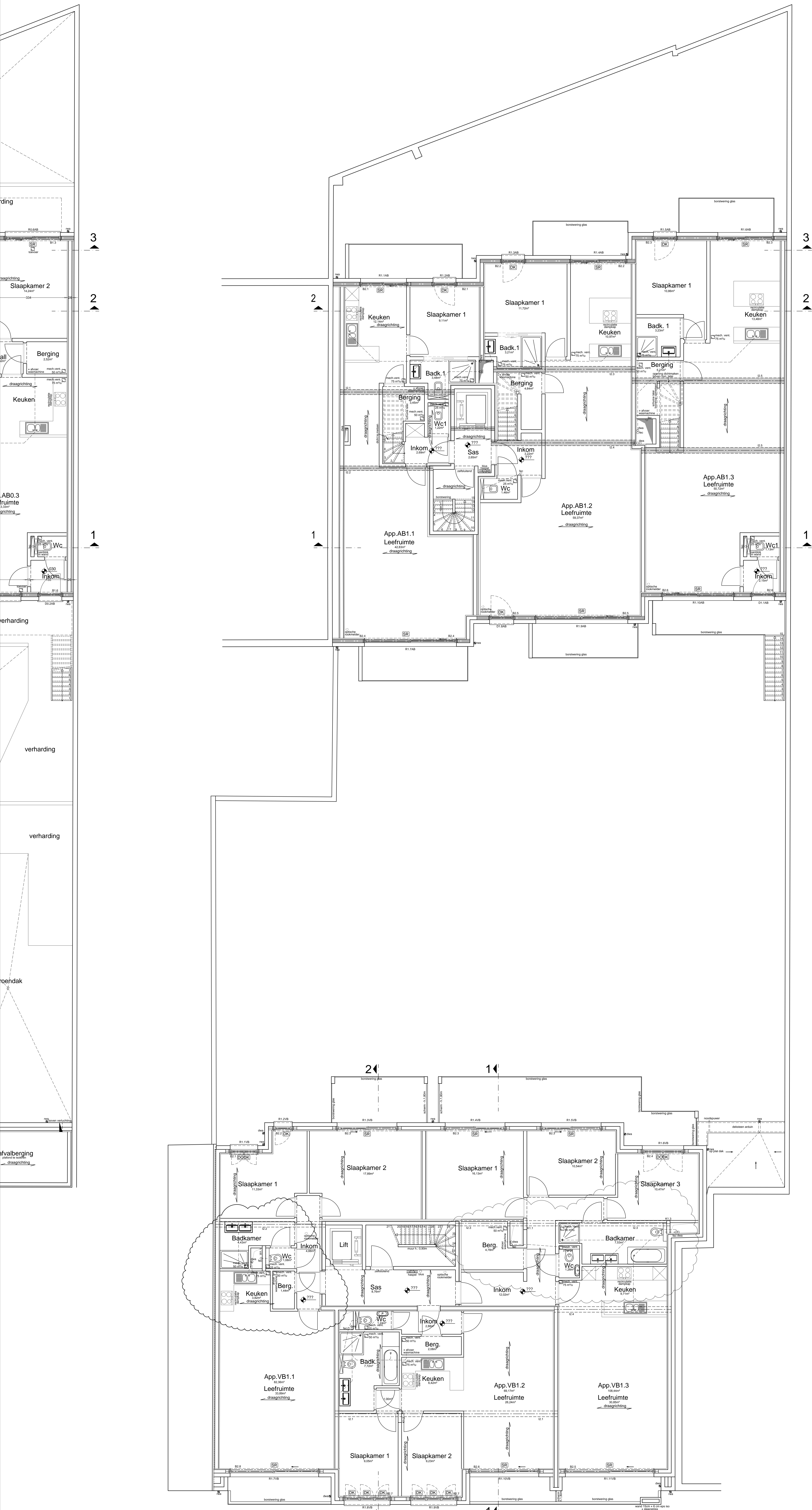
EERSTE VERDIEPING
