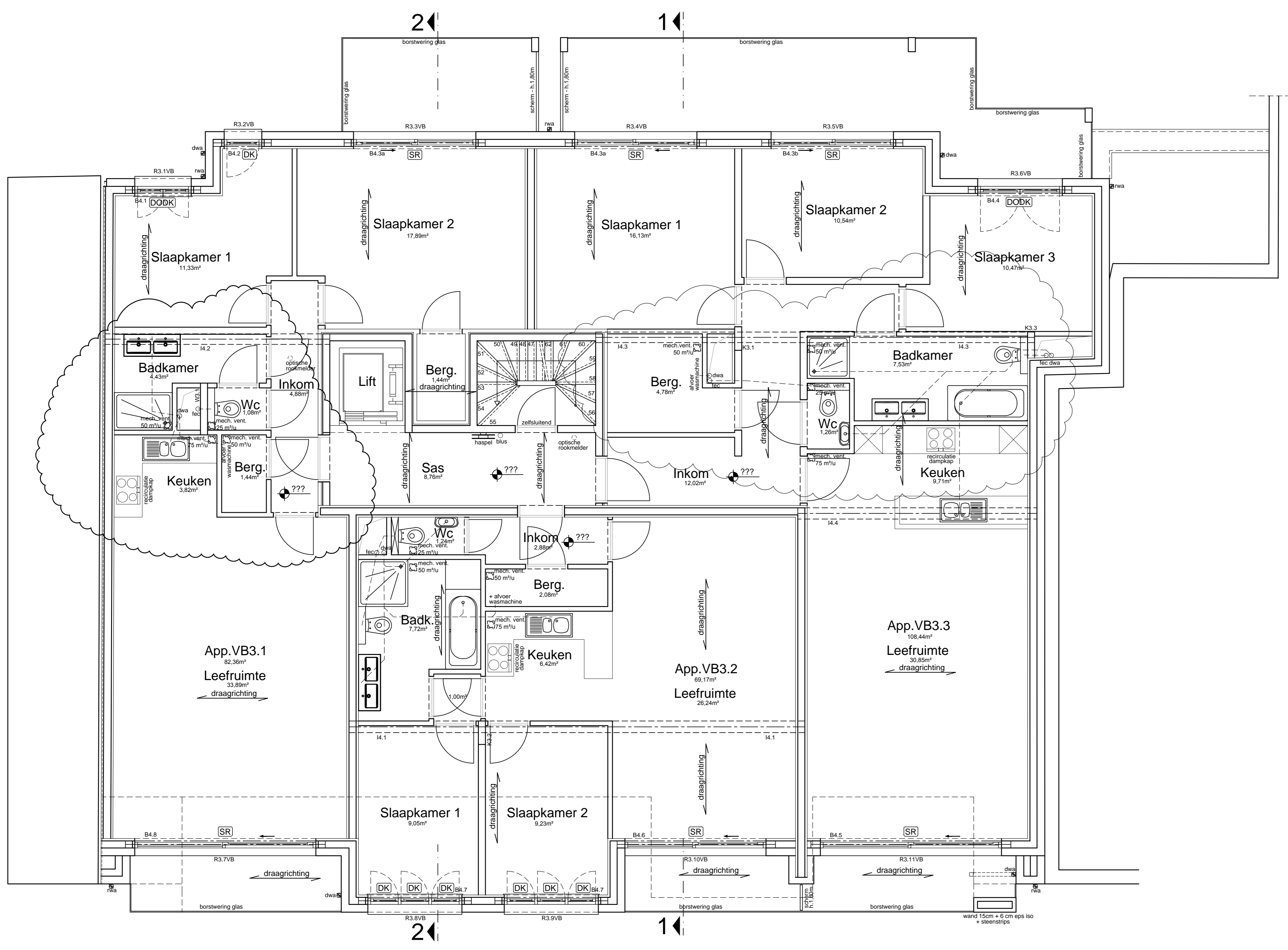
DERDE VERDIEPING
