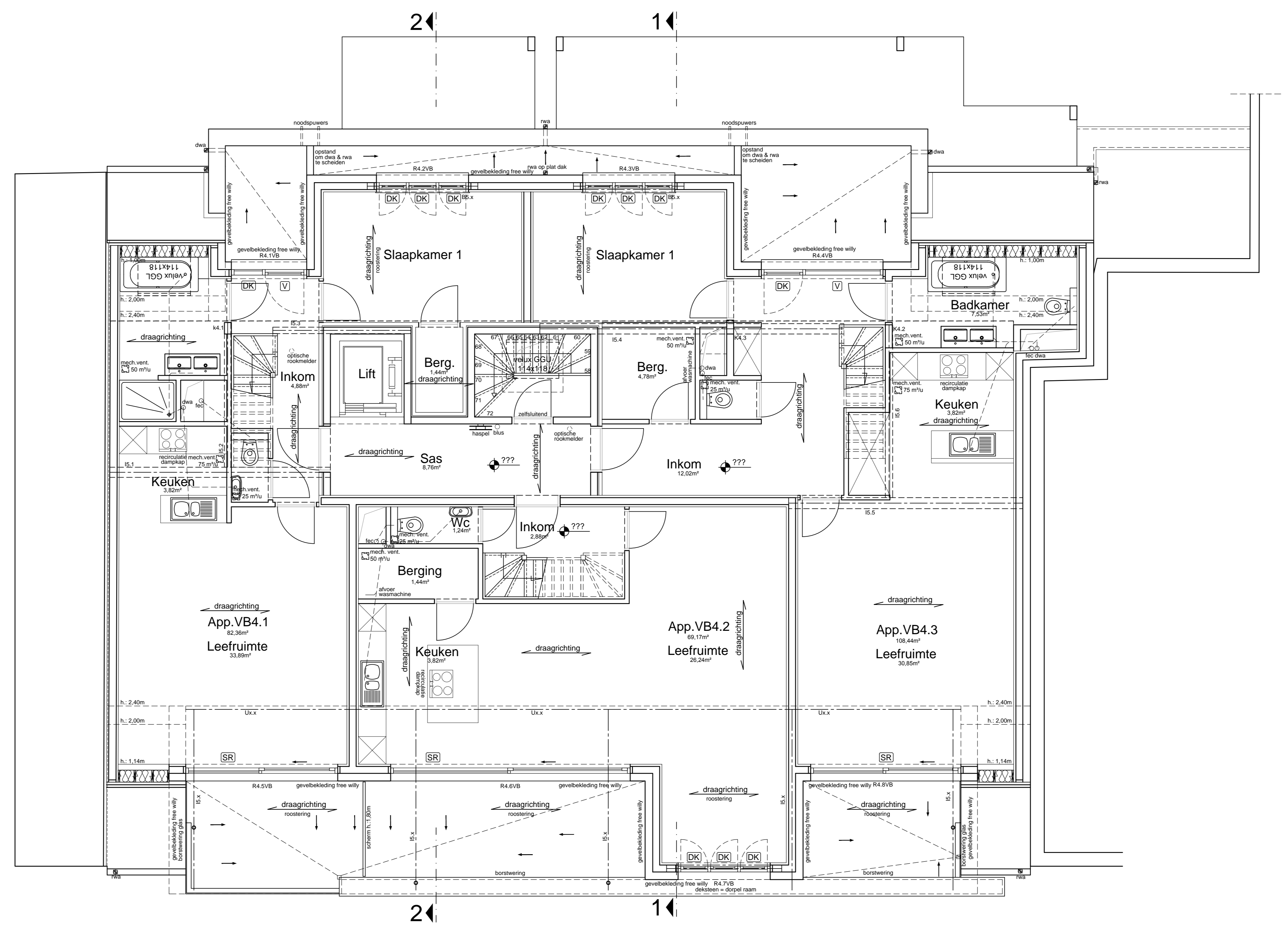
VIERDE VERDIEPING
