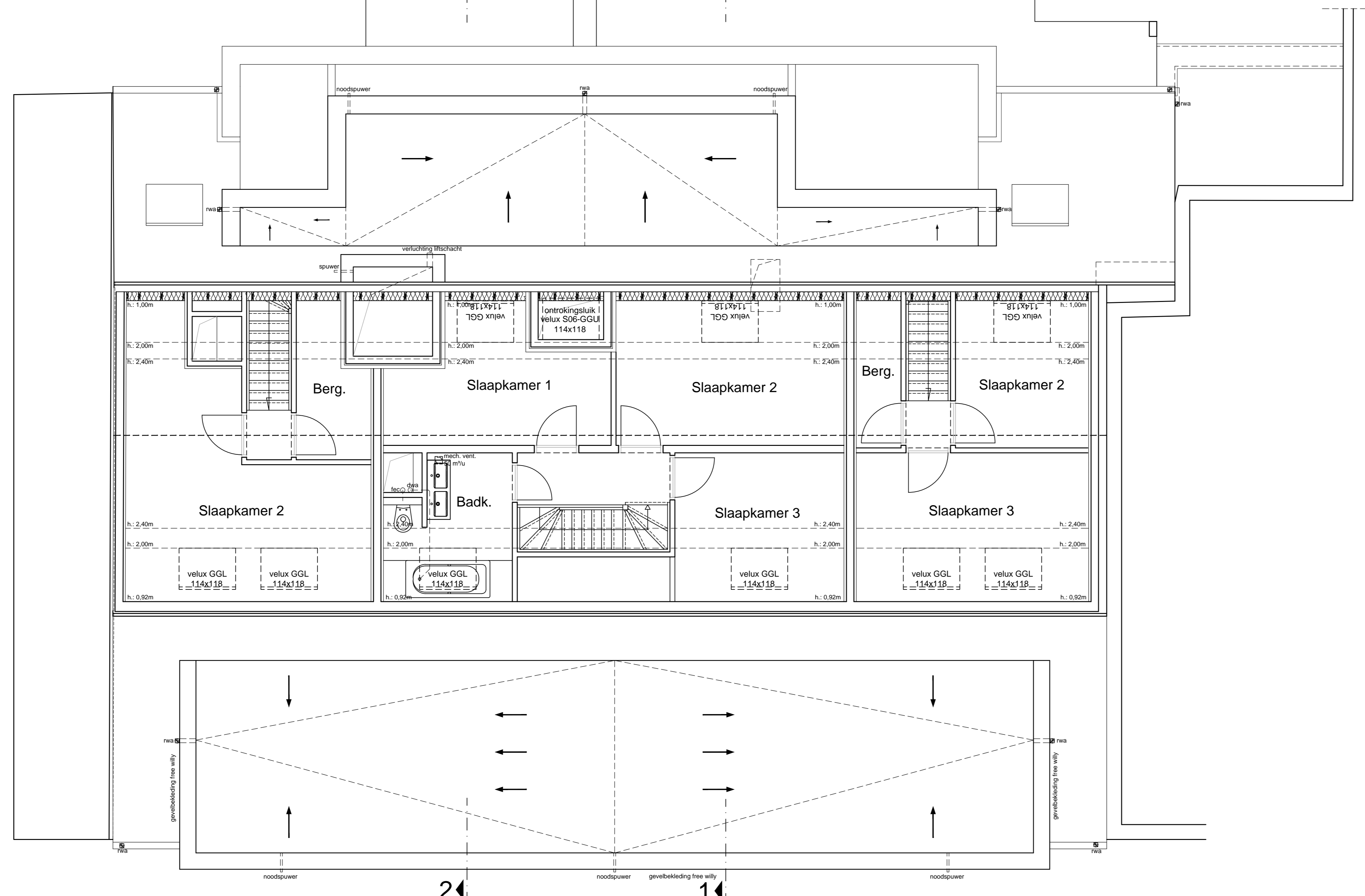
VIJFDE VERDIEPING
